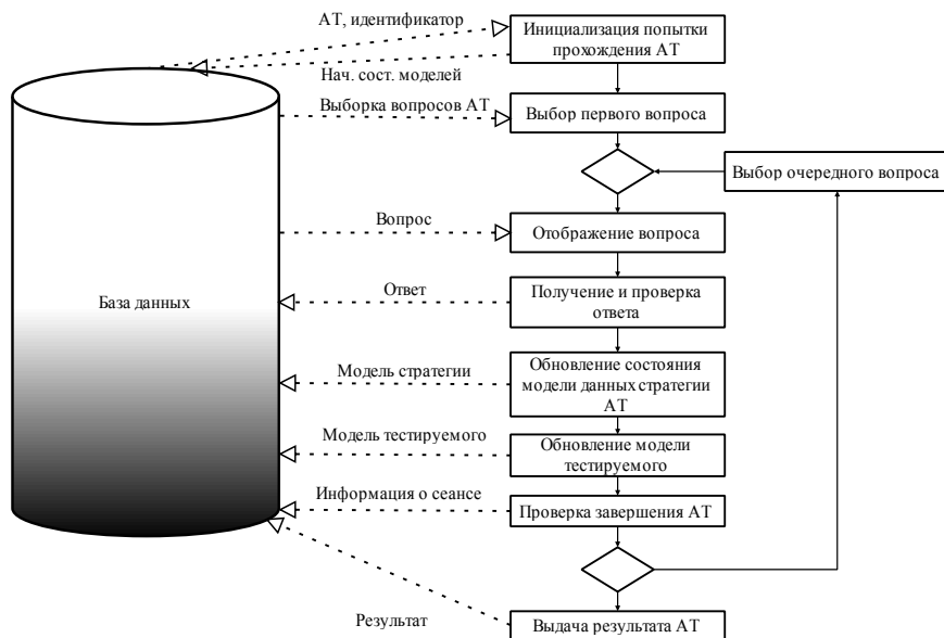
Рис.2 – Алгоритм адаптивного теста
