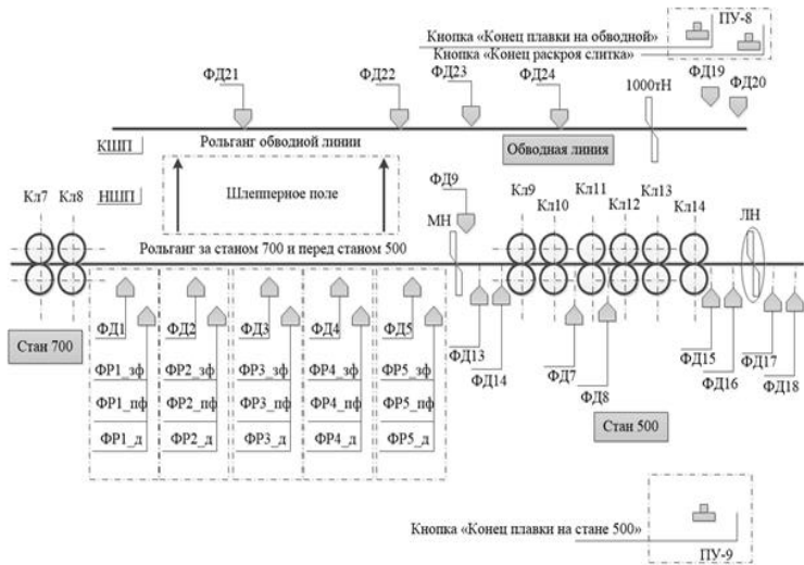
Рис. 1. Структура расположения датчиков сбора первичной информации о состояниях оборудования и параметрах раскраса системы управления раскрасом на ножницах НЗС
