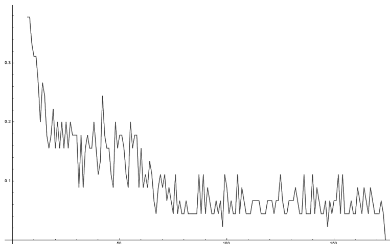
Рисунок 2 – Уменьшение ошибки распознавания в ходе обучения персептрона
