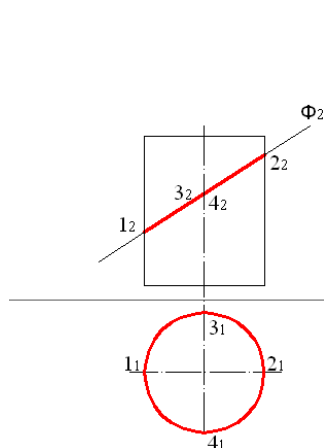
Рис. 1. Первый шаг построения. Построены проекции цилиндра и след фронтально-проецирующей плоскость \Phi_2
