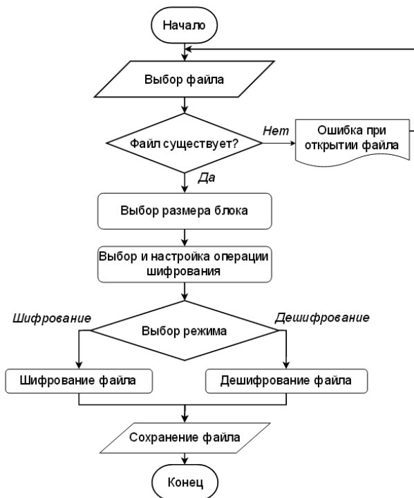
Рисунок 3 – Общий алгоритм работы приложения
