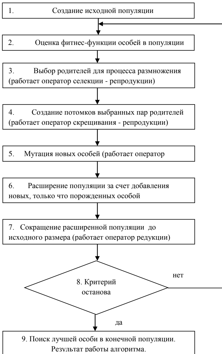
Рисунок 1. Простой генетический алгоритм
