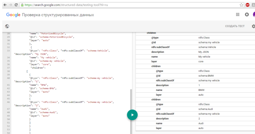
Рисунок 1 – Интерфейс гугл-валидатора
