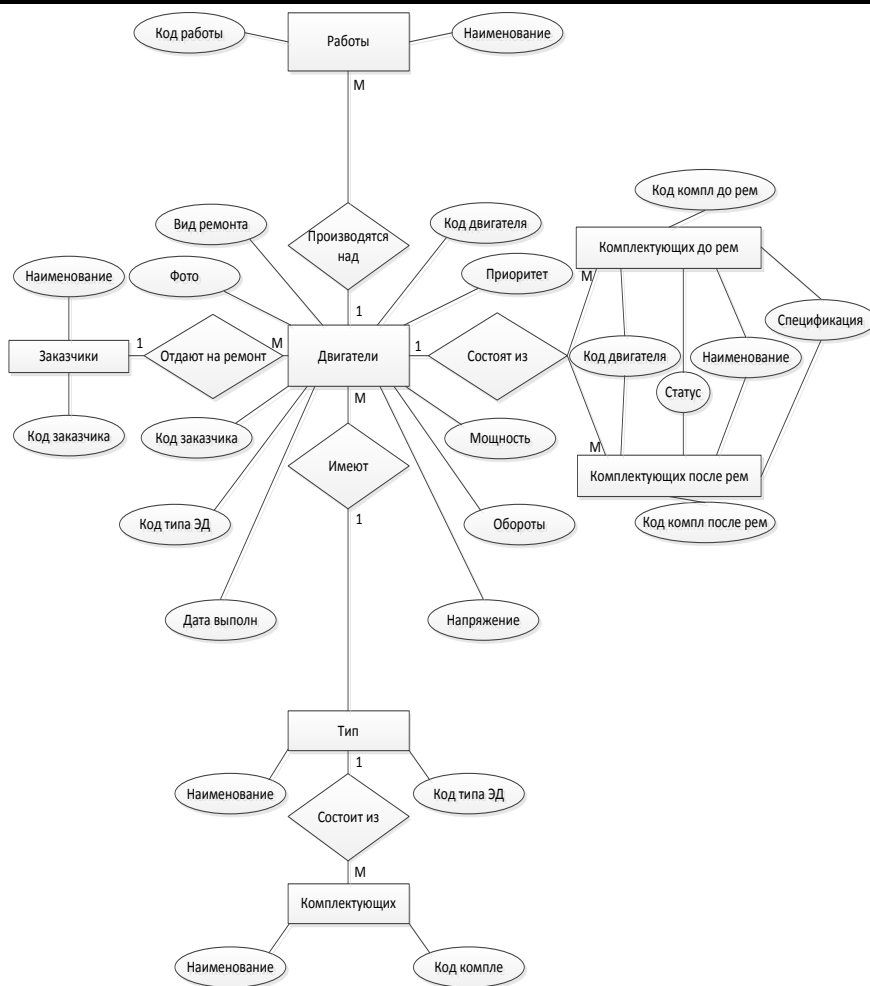
Рисунок 1 – Концептуальная модель
