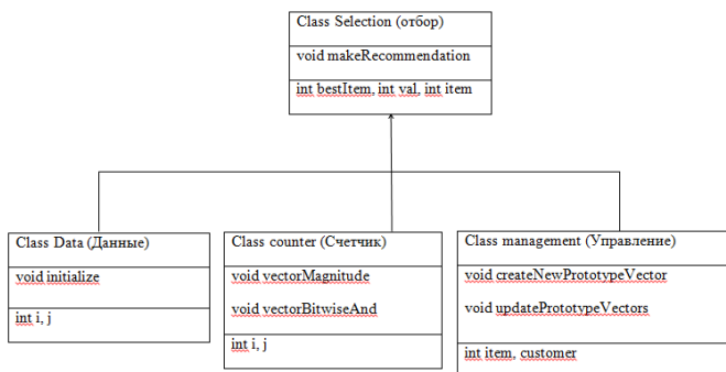
Рис. 1. Диаграмма классов
