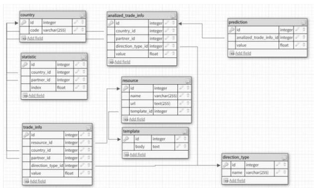
Рисунок 4 – Структура БД
