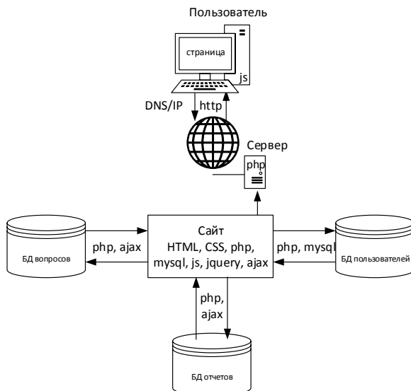
Рисунок 1 – Структура проекта
