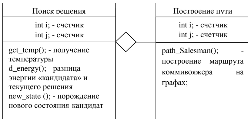
Рисунок 1 – Диаграмма классов
