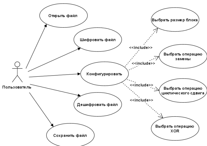
Рисунок 2 – Диаграмма прецедентов
