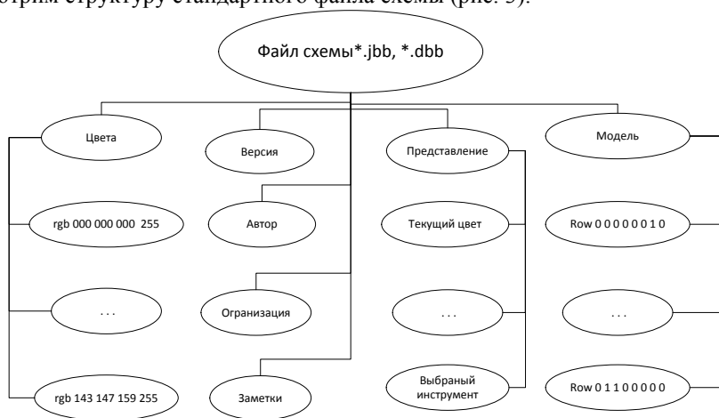
Рисунок 3 – Структура файла
