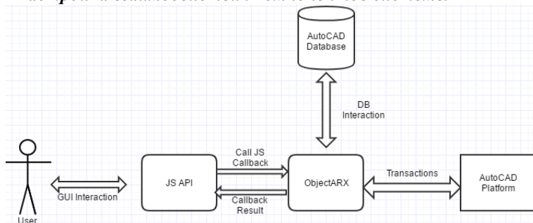
Рисунок 8 – Схема взаимодействия
