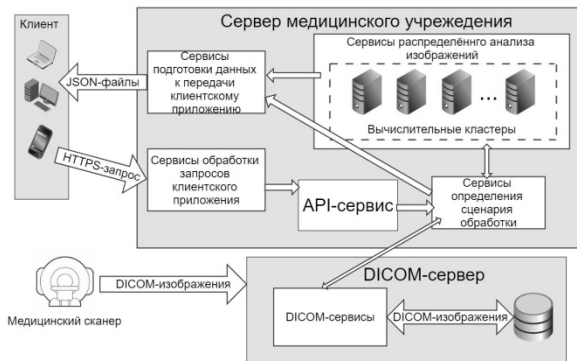
Рисунок 2 – Подробная архитектура подсистемы
