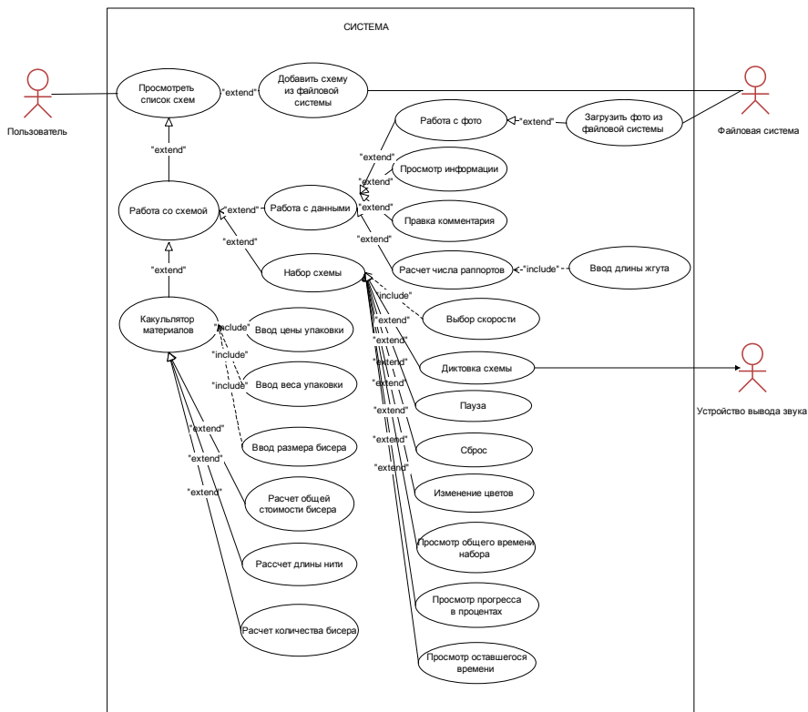
Рисунок 1 – Диаграмма прецедентов
