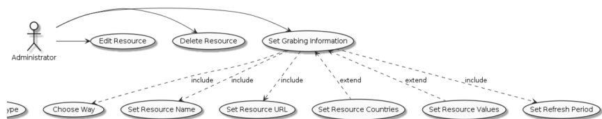
Рисунок 3 – Прецеденты администратора
