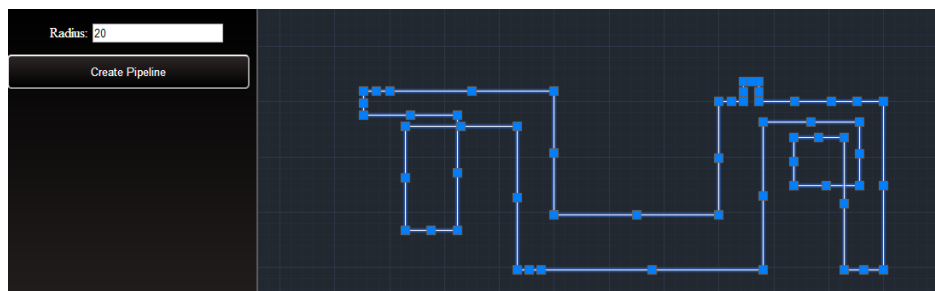
Рисунок 16 – Выделенный контур
